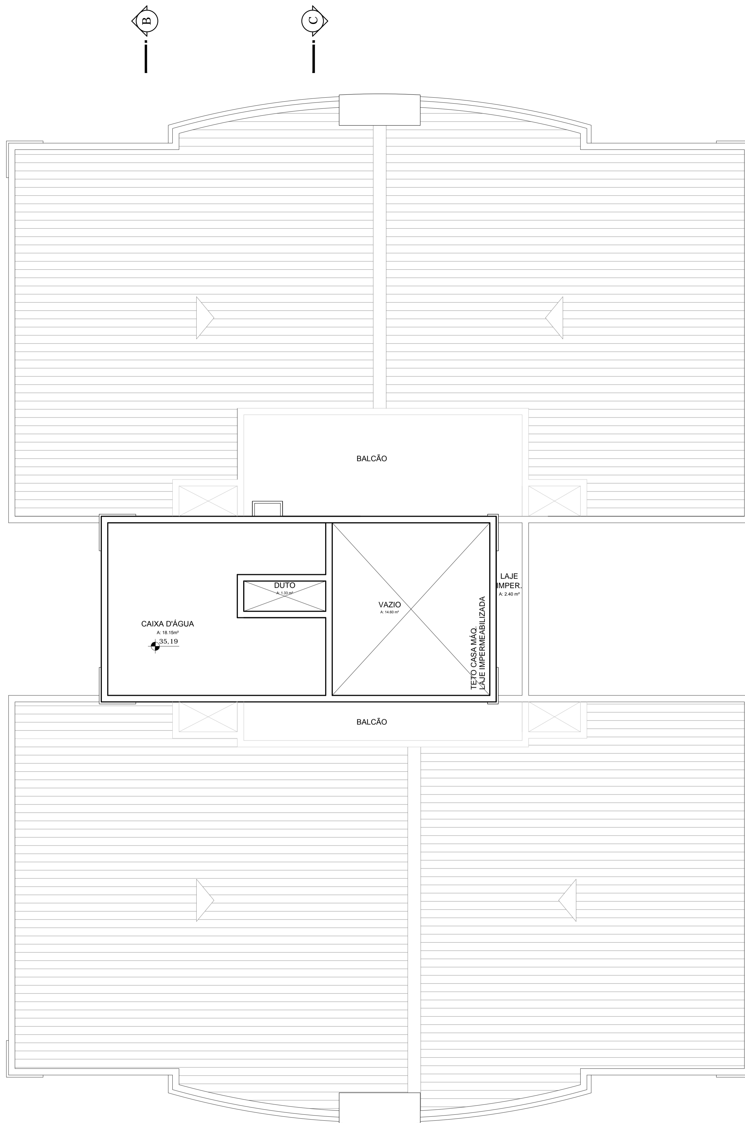
PLANTA BAIXA PAVTO CAIXA D'ÁGUA - TORRE 03/ 04/ 05/ 06/11/ 12 ÁREA DO PAVTO: 24,74m²
